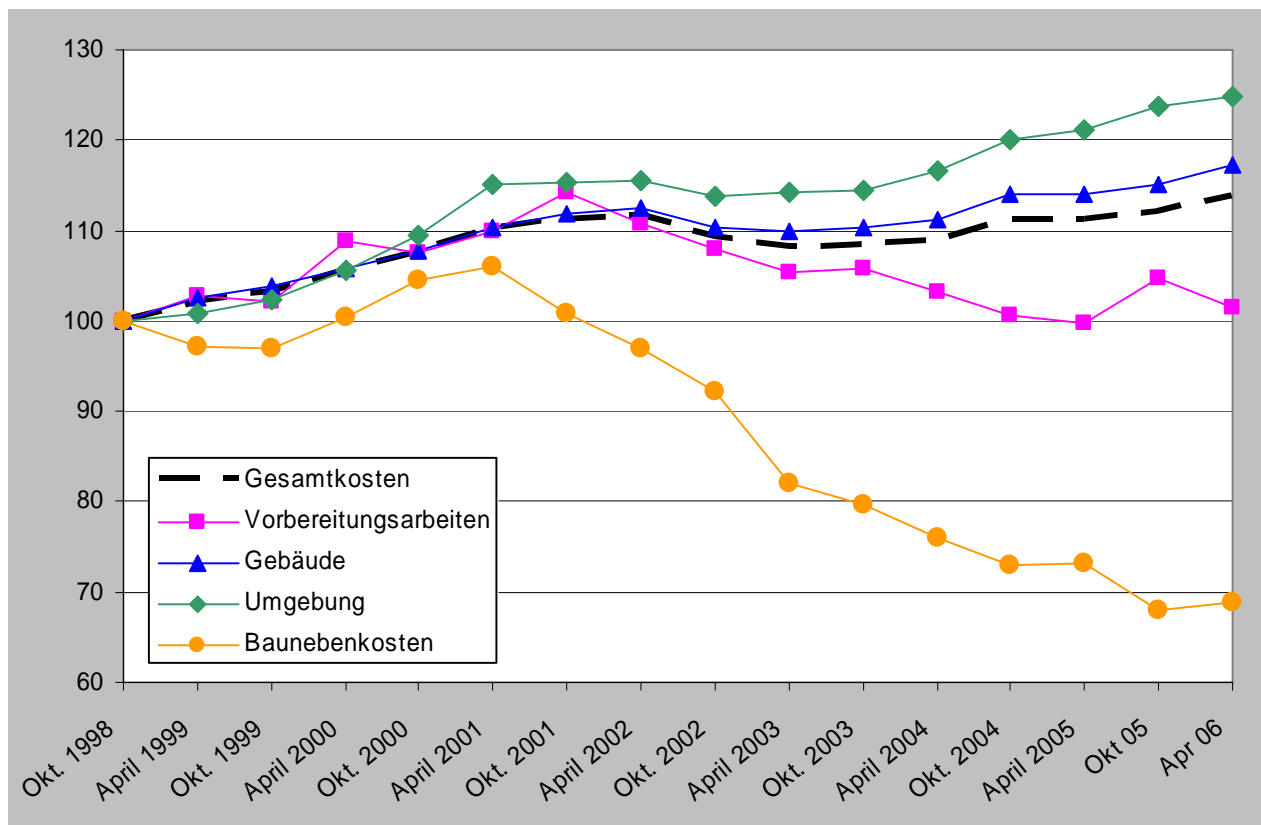
Grafik 2: Baupreisindex nach Hauptgruppen Neubau Mehrfamilienhaus – Espace Mittelland (Basis: Oktober 1998=100)
