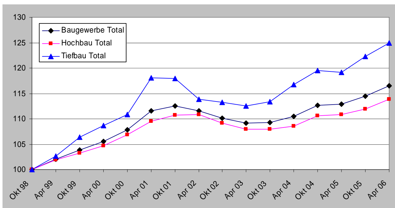
Grafik 4: Entwicklung des Baupreisindexes nach Hoch- und Tiefbau für den Espace Mittelland (Basis: Oktober 1998=100)
