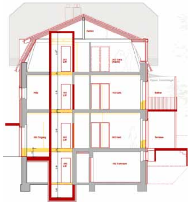
Der Querschnitt zeigt den neuen Lift sowie die neuen Zugänge zum Aussenraum im Erdgeschoss. (Rot: Neu | Gelb: Abbruch)
