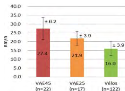
Durchschnittliche punktuelle Geschwindigkeiten in der Steigung (Quelle Grafiken: SVI Merkblatt 2022/01)
