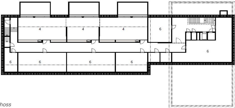
Untergeschoss
