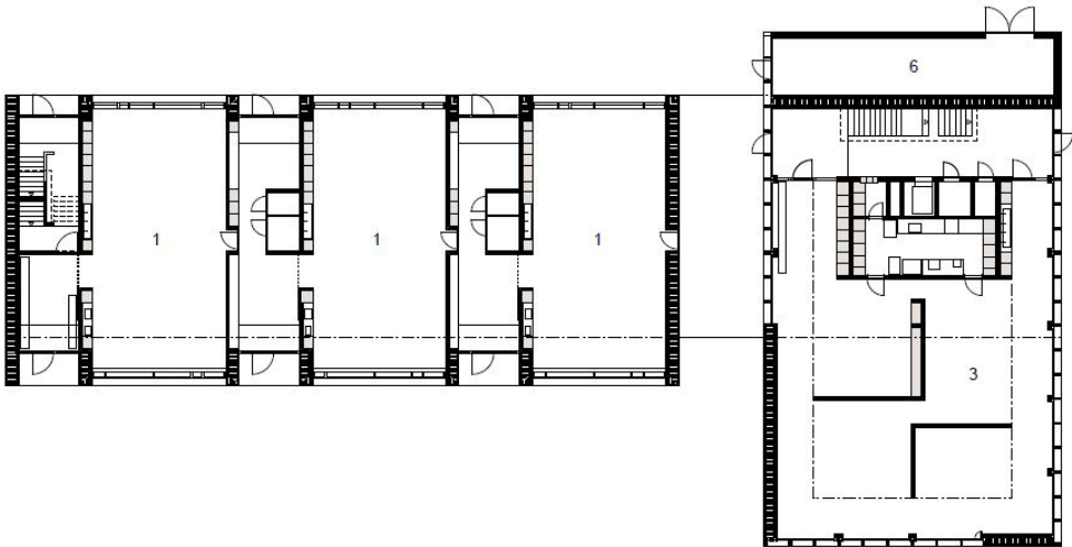
Erdgeschoss
