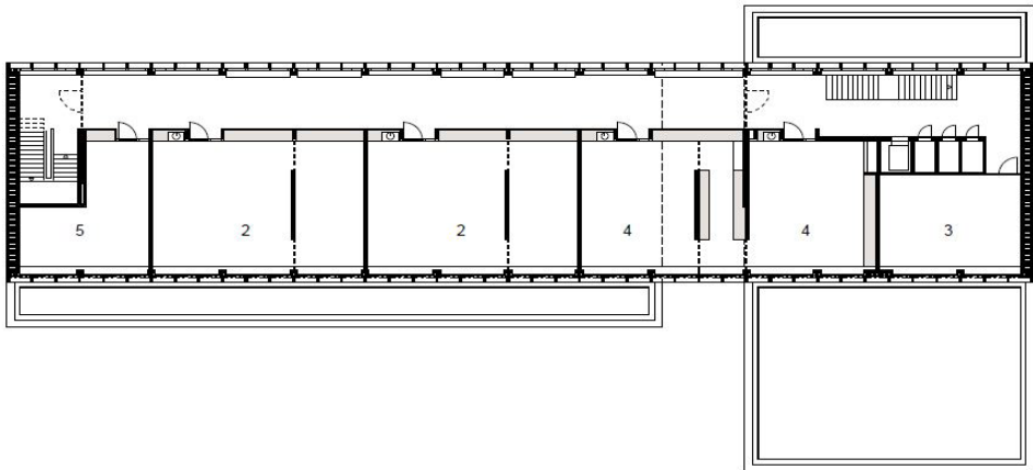
Obergeschoss
