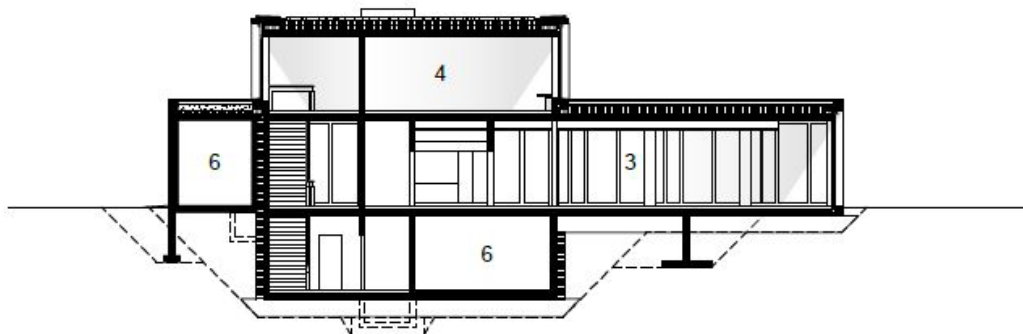
Querschnitt Tagesschule
