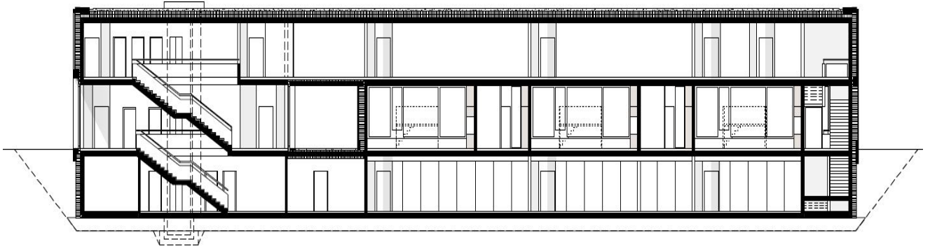
Längsschnitt
