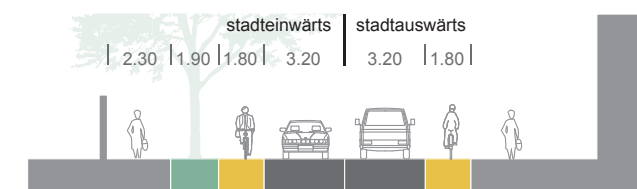
Querschnitt Standstrasse
