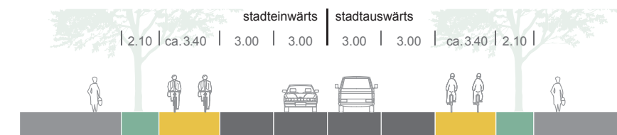
Querschnitt Winkelriedstrasse
