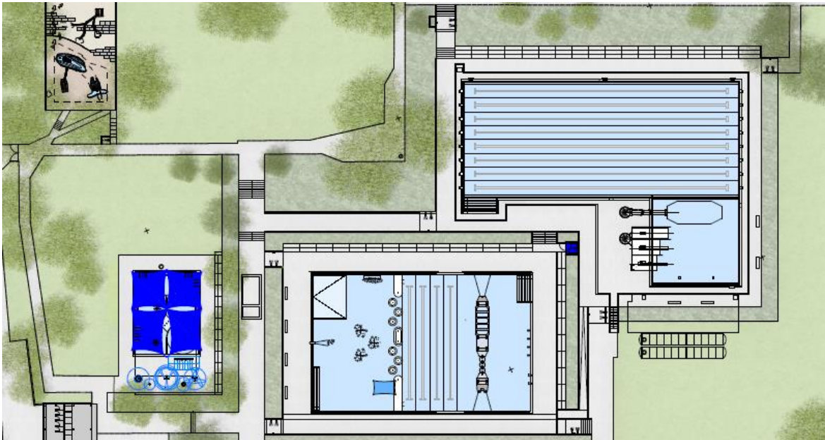
Abb. 11: Situationsplan Sanierungsprojekt
