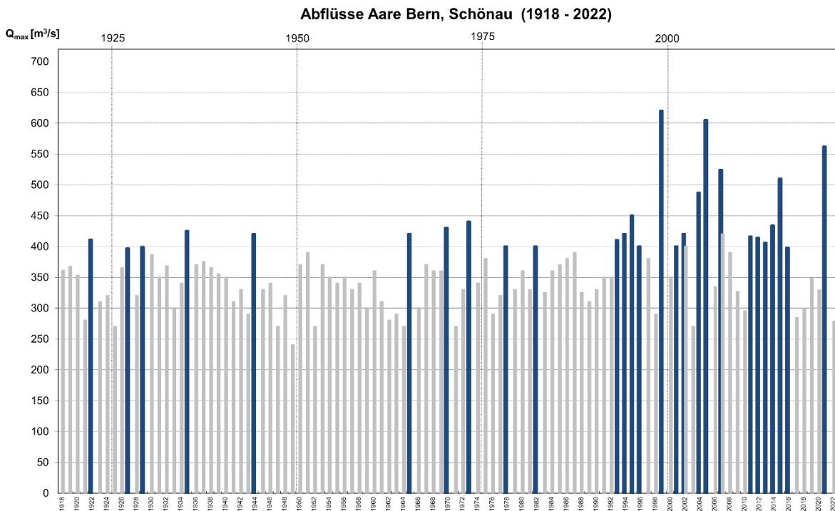
Abbildung Nr. 5: Maximale jährliche Abflussmengen bei der Messtelle Schönau. Die Schadensgrenze liegt bei 400 m³/s. Die blauen Balken stellen Abflussmengen grösser als 400 m³/s dar. In den letzten 25 Jahren ist eine deutliche Häufung solcher Werte festzustellen.
