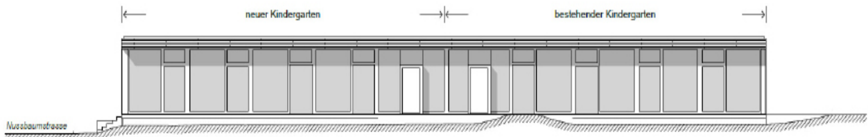
Ansicht Westfassade
