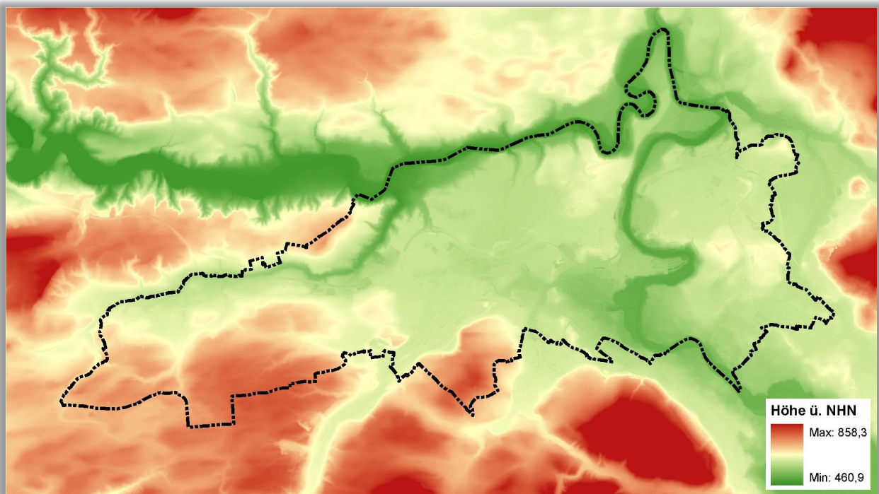
Abb. 2.3: Geländehöhe im Modellierungsgebiet
