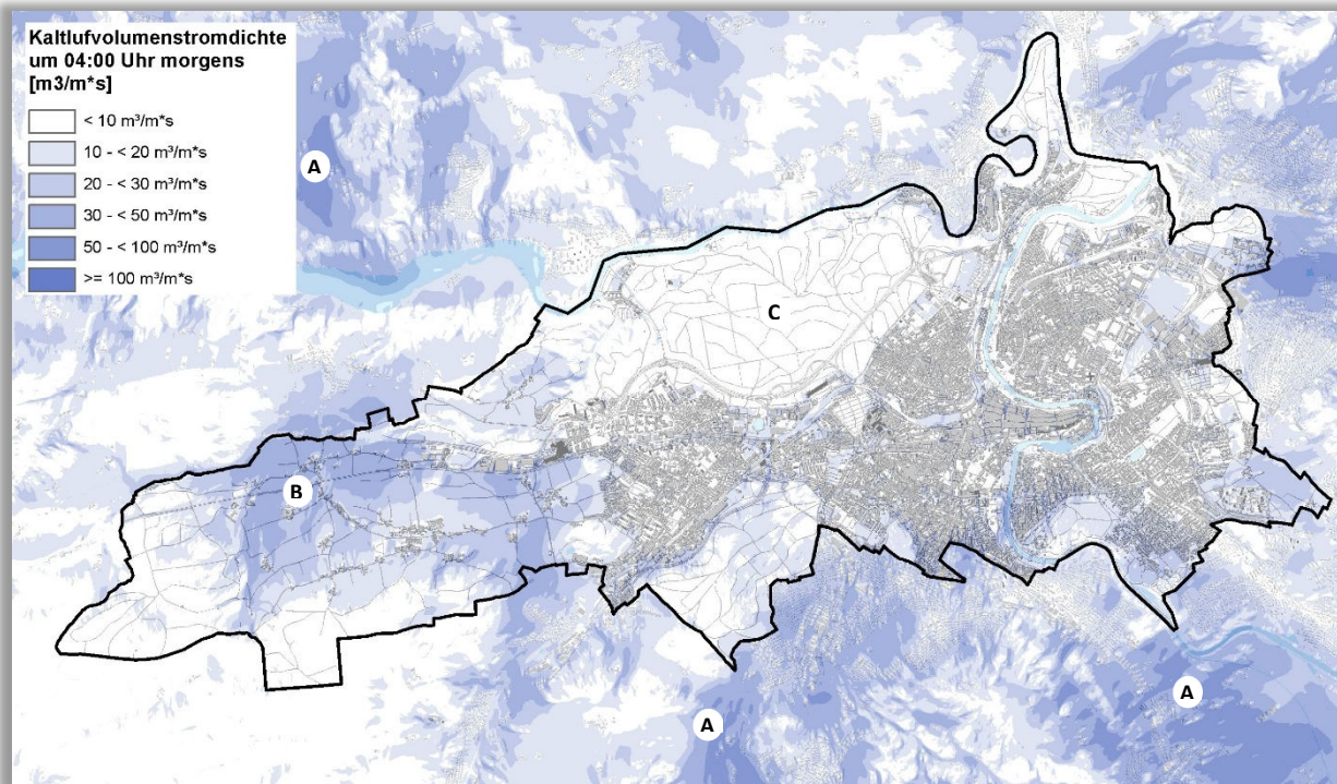
Abb. 4.9: Kaltluftvolumenstrom Gegenwart im Modellgebiet zum Zeitpunkt 4 Uhr morgens
