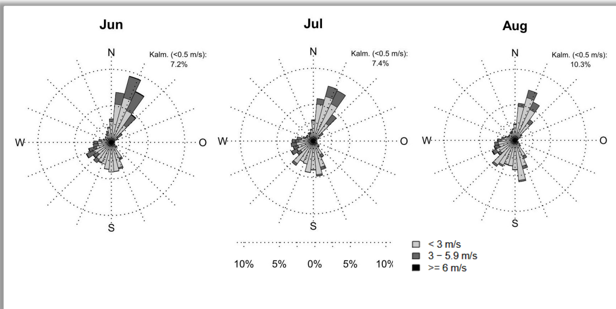
Abb. 3.7: Windrosen der Station Bern/Zollikofen 365 m ü.M. für die Sommermonate Juni, Juli und August (Quelle: Meteoschweiz 2020c).
