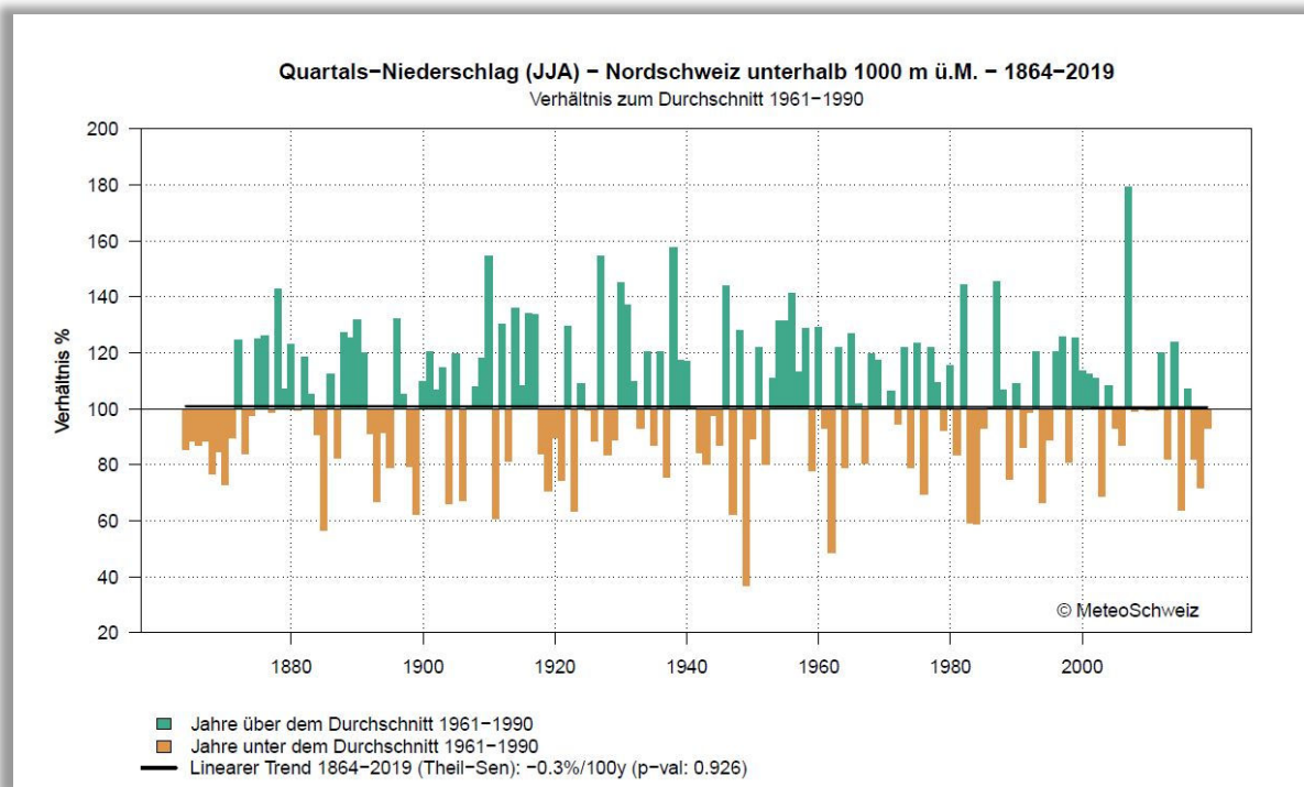
Abb. 3.6: Entwicklung der sommerlichen Niederschlagssummen für die Nordschweiz unter 1.000 m ab 1864 bis heute im Vergleich zur Periode 1961 – 1990 (Quelle: Meteoschweiz 2020d)
