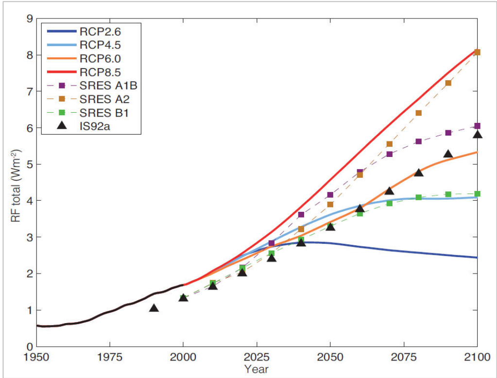
Abb. 3.8: Anthropogener Strahlungsantrieb der verschiedenen IPCC-Klimaszenarien (die schwarze Linie repräsentiert Messwerte; Cubasch et al. 2013)
