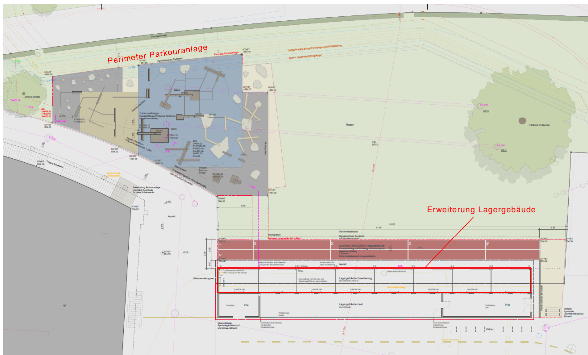
Situationsplan Vorprojekt für die Parkouranlage und Erweiterung des Lagergebäudes Sportplatz Wankdorf. (Quelle; Müller Wildbolz Partner GmbH)
