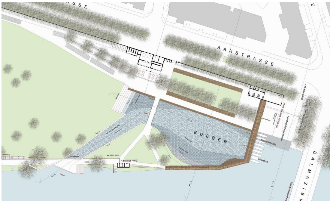
Sanierungsprojekt Bueberseeli (genordete Plandarstellung ohne Massstab)
