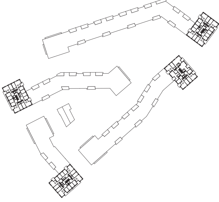
5. OBERGESCHOSS 1:500
