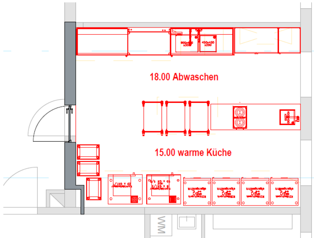
Grundriss Vorprojekt Regenerationsküche TS Türlmä (ProCulina GmbH)
