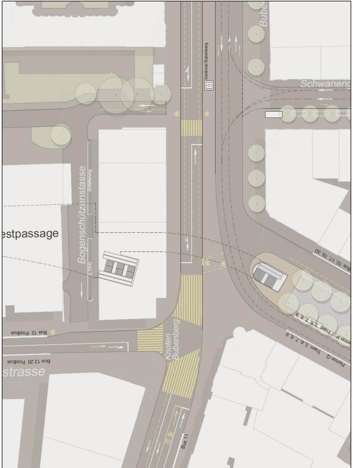
Betriebs- und Gestaltungskonzept 2015: Variante 1 mit ergänzender Unterführung und Denkmal auf dem Bubenbergrastplatz
