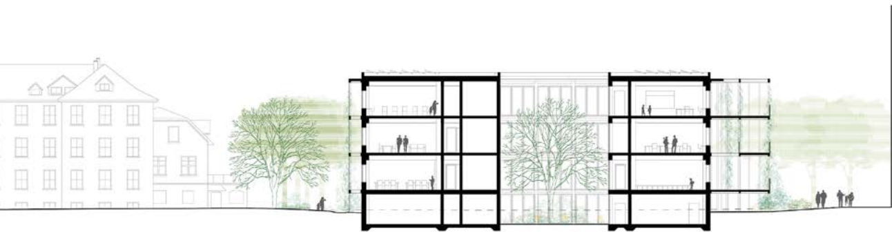
Schnitt B-B
