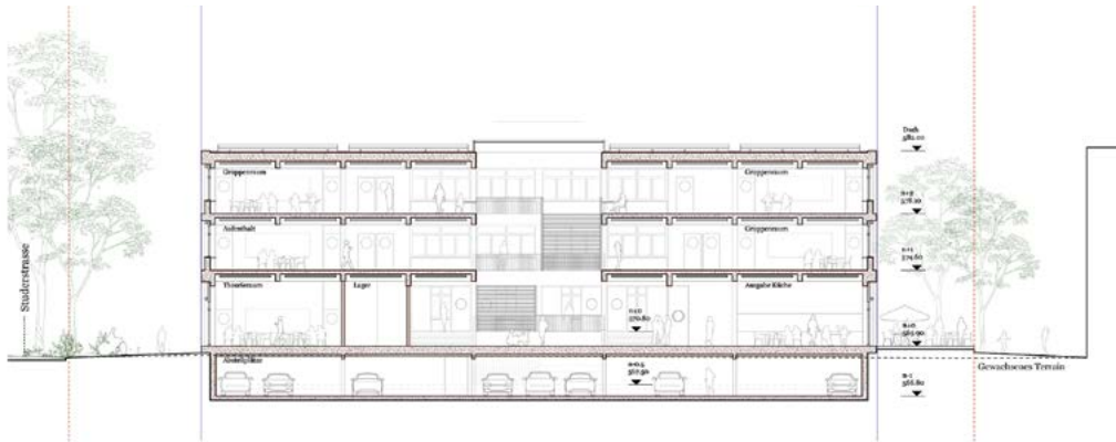
Querschnitt Schule
