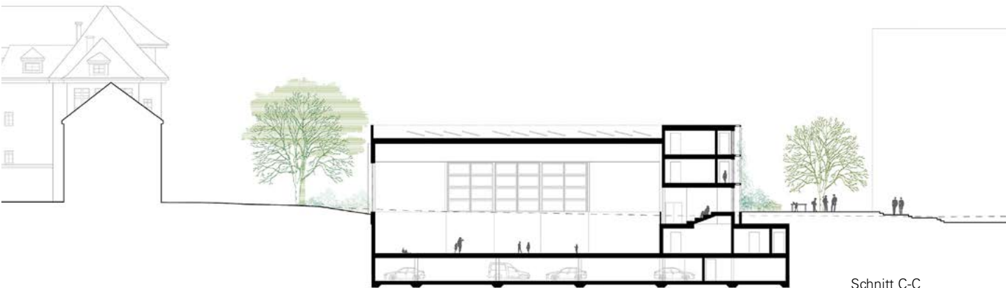
Schnitt C-C
