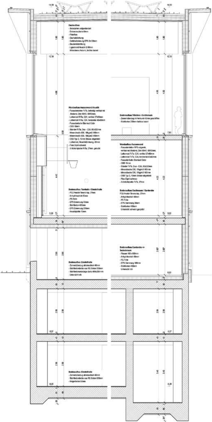
Detailschnitt Turnhalle
