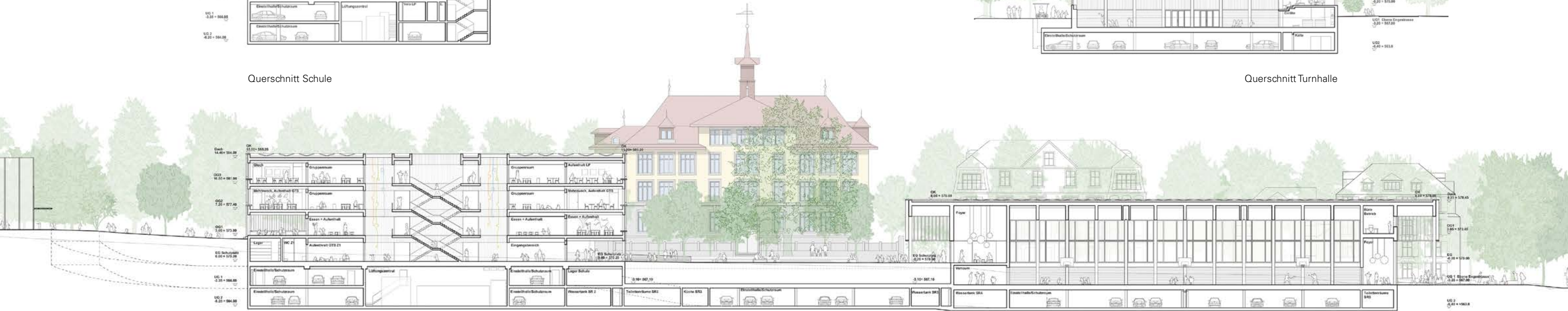
Längsschnitt
