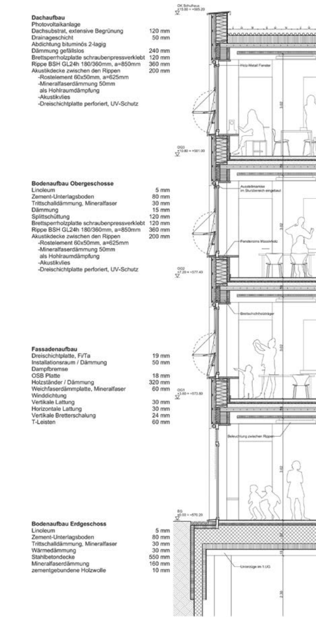
Detailschnitt Schule
