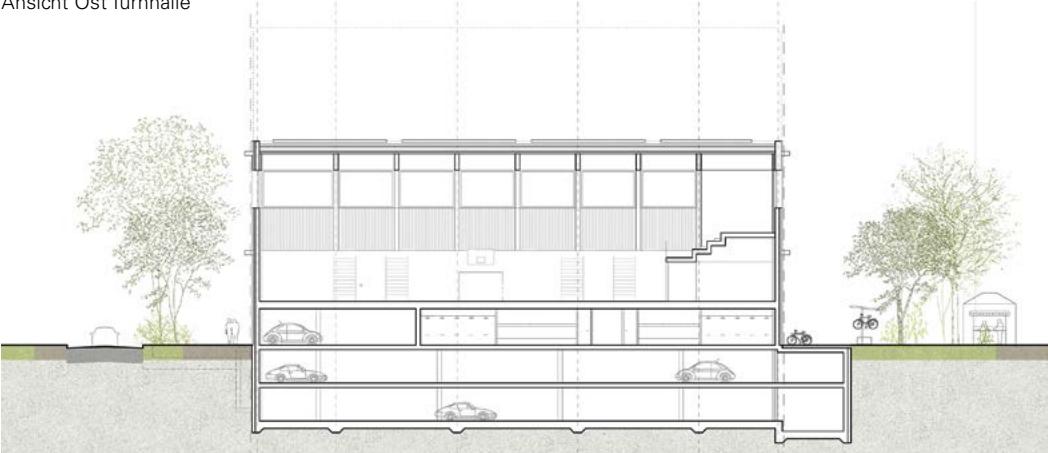
Querschnitt Turnhalle
