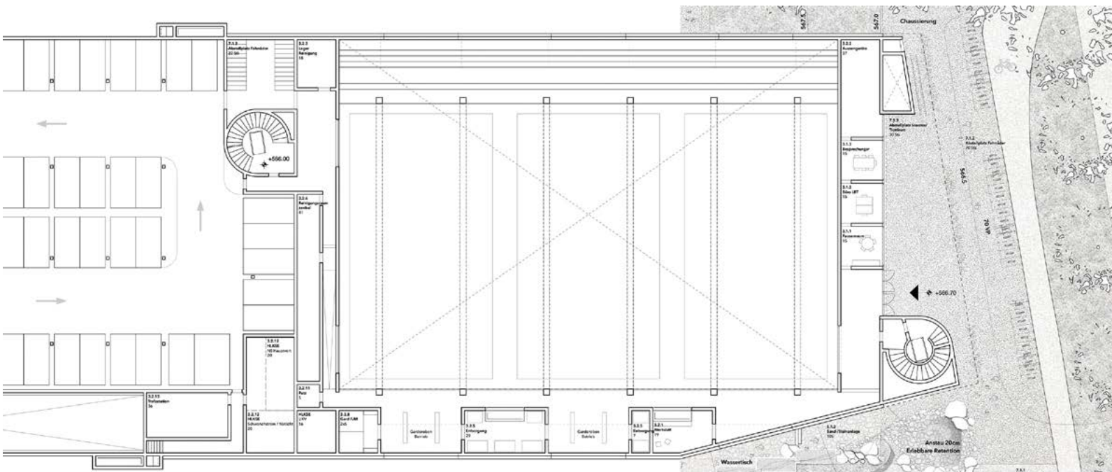
Grundriss 1. Untergeschoss
