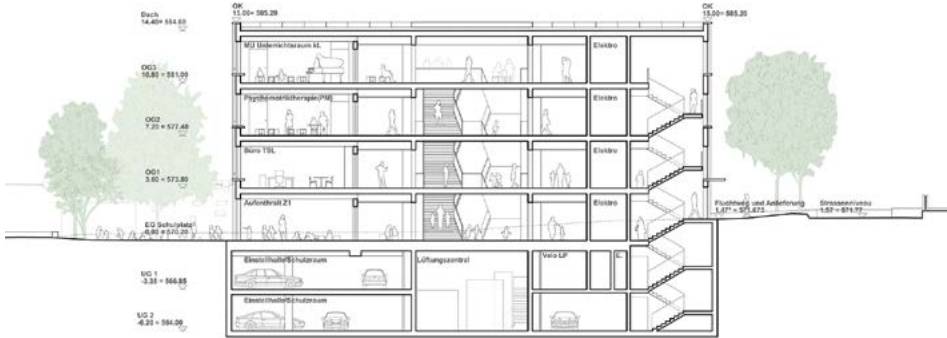
Querschnitt Schule
