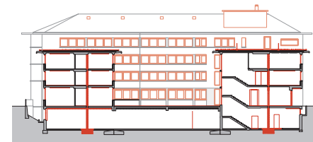
Querschnitt West-/Ostflügel
