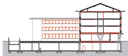
Querschnitt Nordflügel
