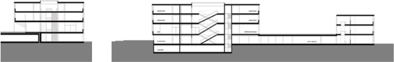
Querschnitt Primarschule
