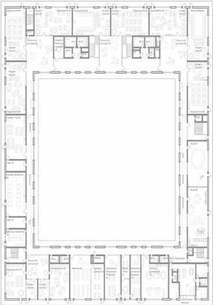
Grundriss Obergeschoss
