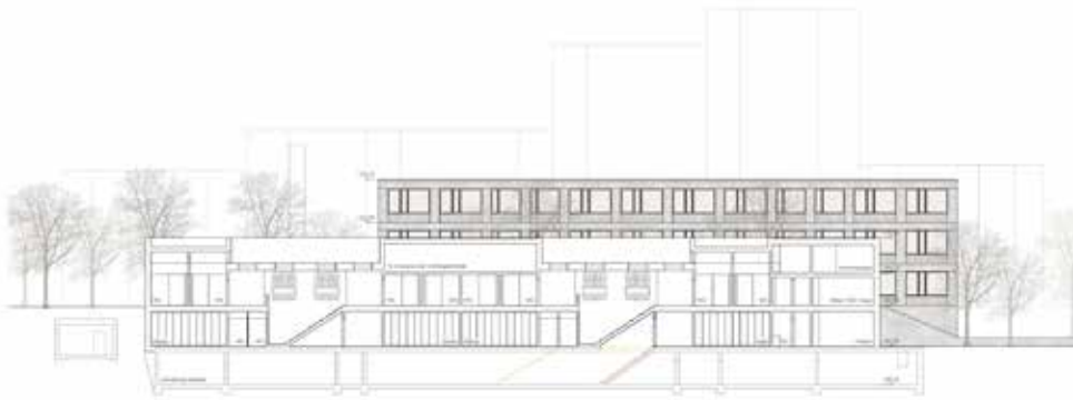
Schnitt D-D, Längsschnitt Basisstufe
