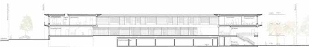
Schnitt BB
