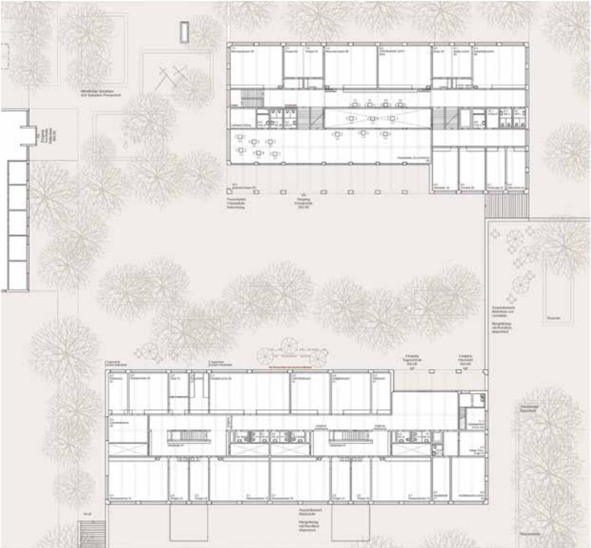
Grundriss Erdgeschoss
