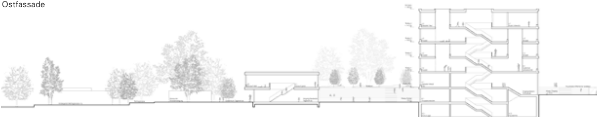
Schnitt A-A
