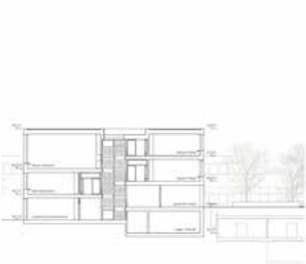
Querschnitt C-C, Primarstufe
