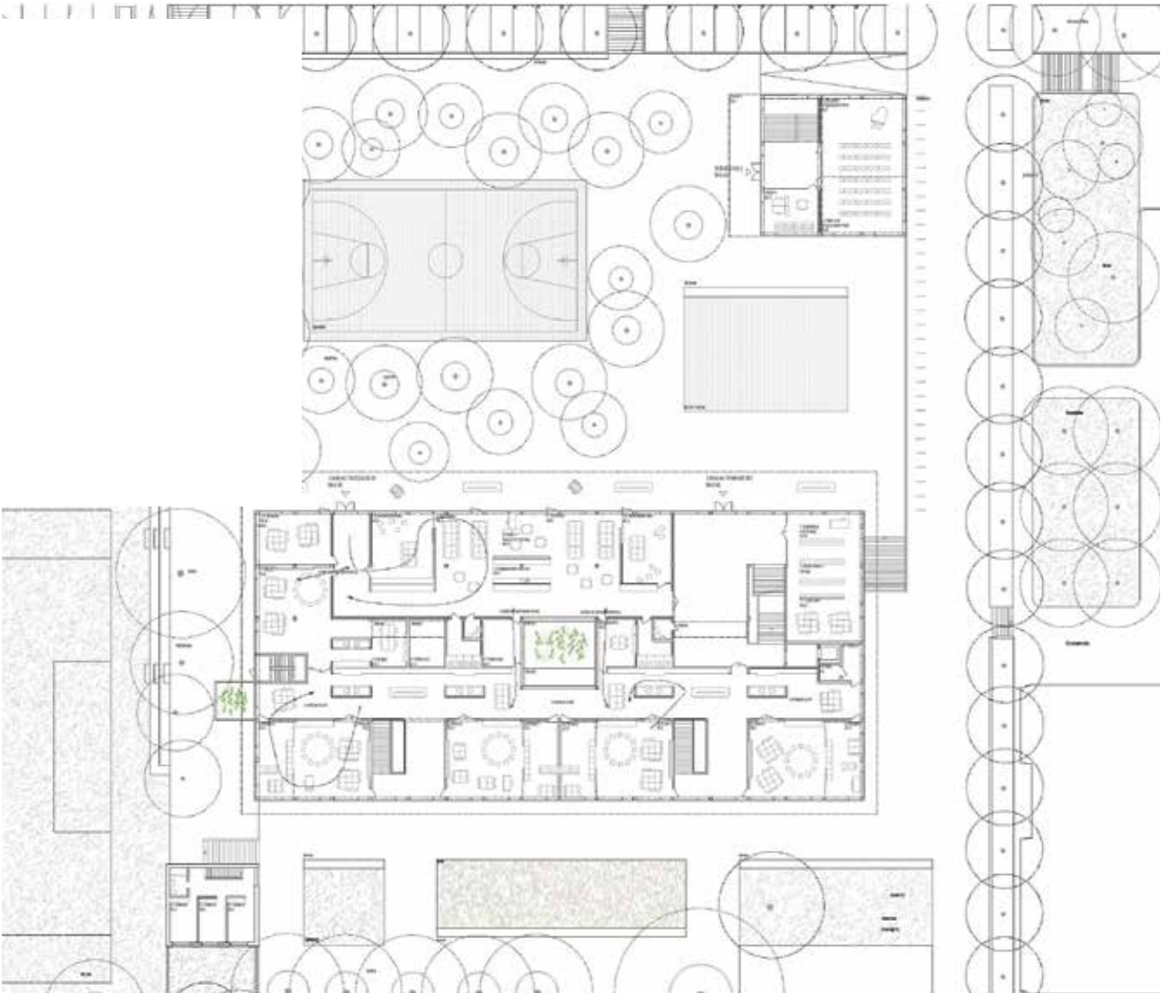
Grundriss Erdgeschoss
