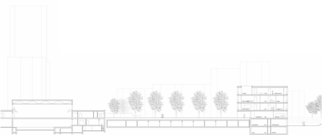
Längsschnitt
