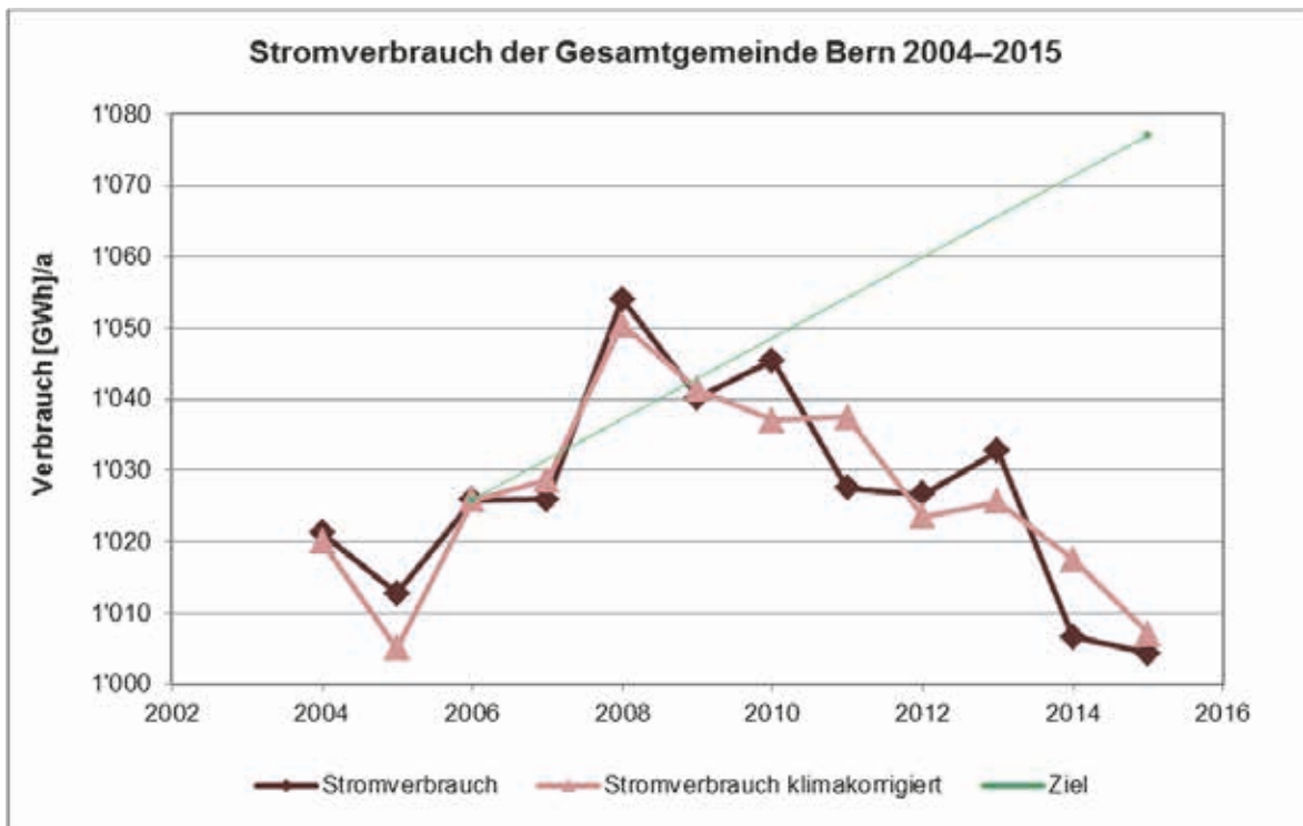
Abbildung 28: Zeitliche Entwicklung des Stromverbrauchs der Gesamtgemeinde Bern im Vergleich mit dem Ziel aus der Energiestrategie (Quelle: ewb) Hinweis: y-Achse beginnt bei 1000 GWh/a.
