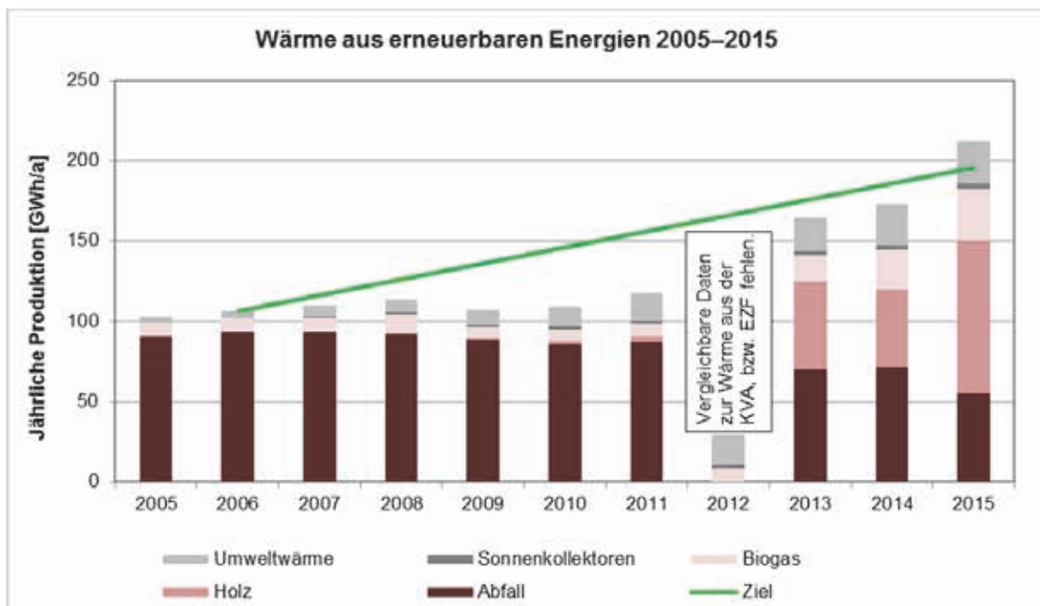
Abbildung 31: Produktion von Wärme aus erneuerbaren Energien. Zeitliche Entwicklung der Produktion und Vergleich mit dem Zielpfad (Quelle: ewb)
