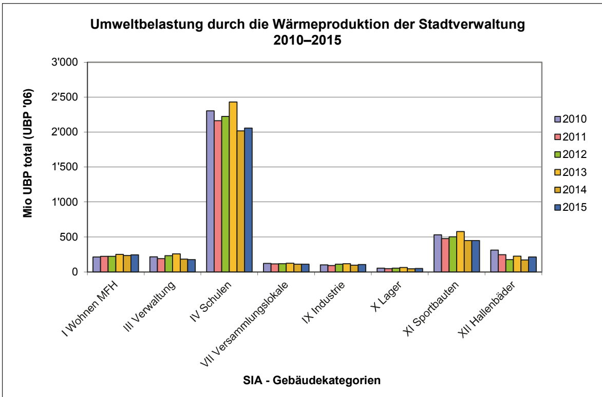
Abbildung 6: Umweltbelastung durch die Wärmeproduktion der Stadtverwaltung nach Gebäudekategorie (Quelle: Immobilien Stadt Bern) NICHT heizgradtagbereinigt
