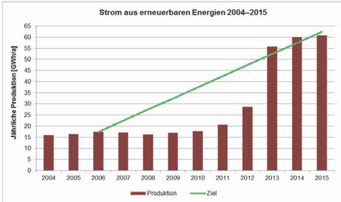
Abbildung 29: Produktion von Strom aus neuen erneuerbaren Energien Zeitliche Entwicklung der Produktion und Vergleich mit dem Zielpfad (Quelle: ewb)
