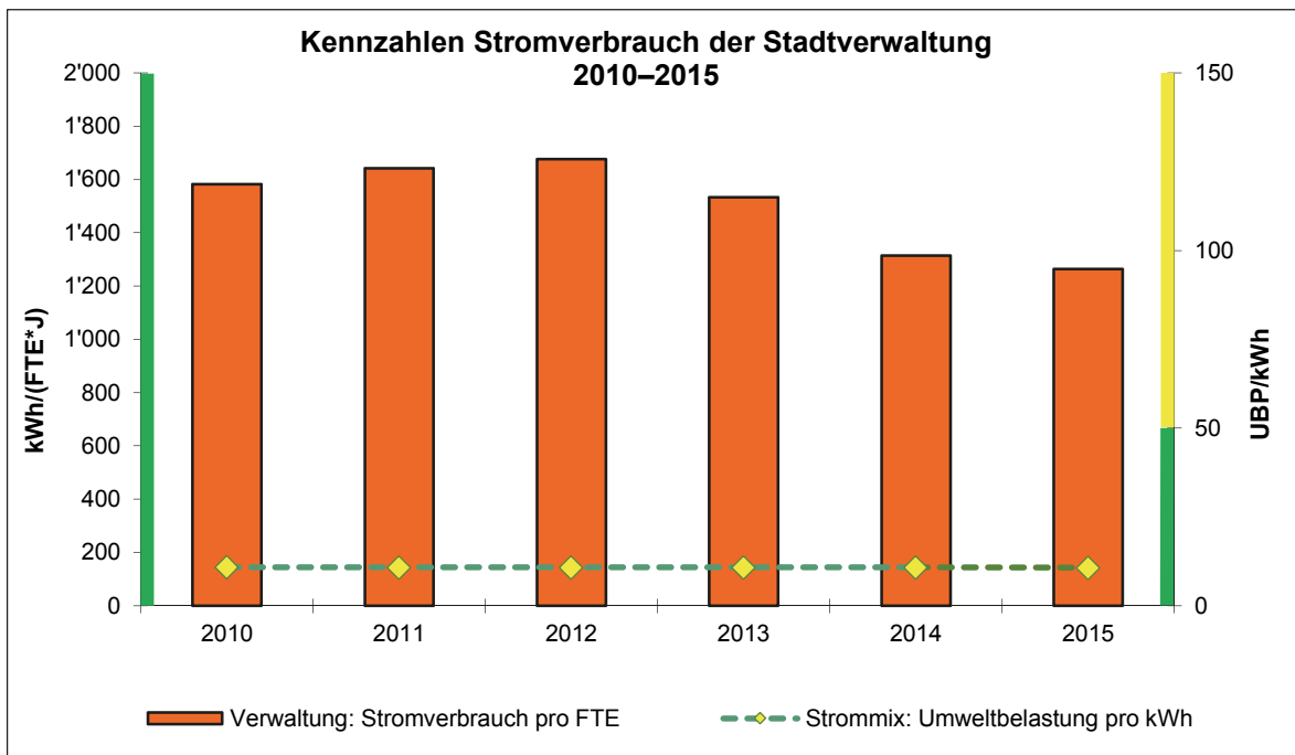
Abbildung 9: Stromverbrauch der Stadtverwaltung pro Vollzeitstelle und durchschnittliche Umweltbelastung pro kWh des verwendeten Strommixes (Quelle: Immobilien Stadt Bern) Die Farbskalen links und rechts dienen dem qualitativen Vergleich mit der Bundesverwaltung und Dienstleistungsbetrieben der Privatwirtschaft: grün = gut, gelb = mittel
