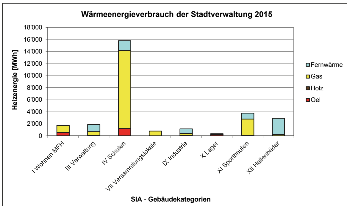
Abbildung 5: Wärmeenergieverbrauch der Stadtverwaltung Bern nach Gebäudekategorie und Energieträger (Quelle: Immobilien Stadt Bern)
