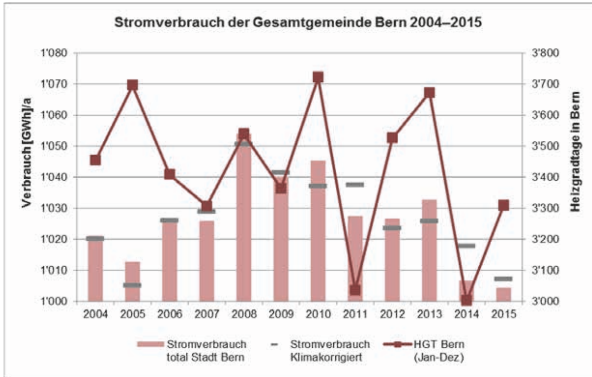
Abbildung 27: Zeitliche Entwicklung des gesamten Stromverbrauchs der Gesamtgemeinde Bern. (Quelle: ewb) Hinweis: y-Achse links beginnt bei 1000 GWh/a, rechts bei 3000 HGT.
