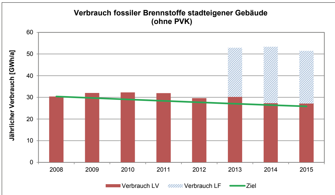
Abbildung 32: Verbrauch fossiler Brennstoffe, klimakorrigiert. Berücksichtigt sind die Gebäude der Immobilien Stadt Bern, Liegenschaften im Verwaltungsvermögen (LV) und Liegenschaften im Finanzvermögen (LF). Als fossile Brennstoffe zählen Erdgas, Heizöl und 50% der Wärme aus Abfällen (Quelle: Immobilien Stadt Bern)
