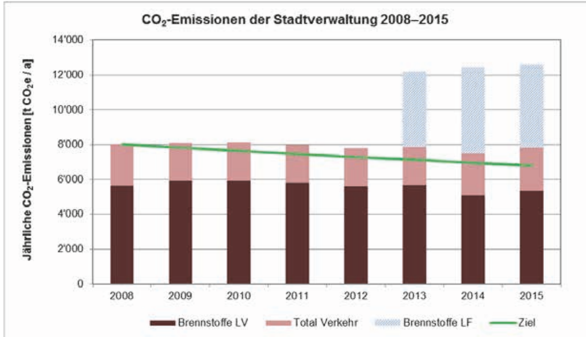
Abbildung 33: CO 2 -Emissionen, klimakorrigiert. Berücksichtigt sind die Heizung der Gebäude der Immobilien Stadt Bern, Liegenschaften im Verwaltungsvermögen (LV) und im Finanzvermögen (LF) und der Verkehr der Verwaltung (inklusive Pendlerverkehr). Die Wärme aus dem Kehricht wird hier als CO 2 -neutral betrachtet (s. Text).
