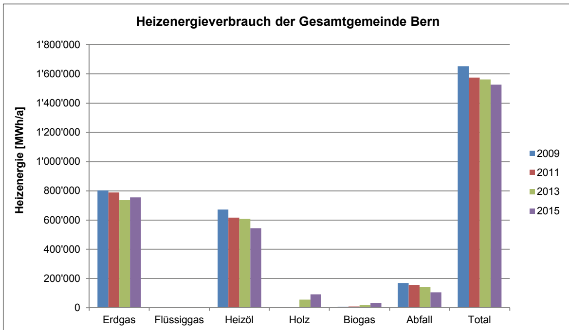
Abbildung 18: Heizenergieverbrauch der Gesamtgemeinde Bern nach Energieträgern
