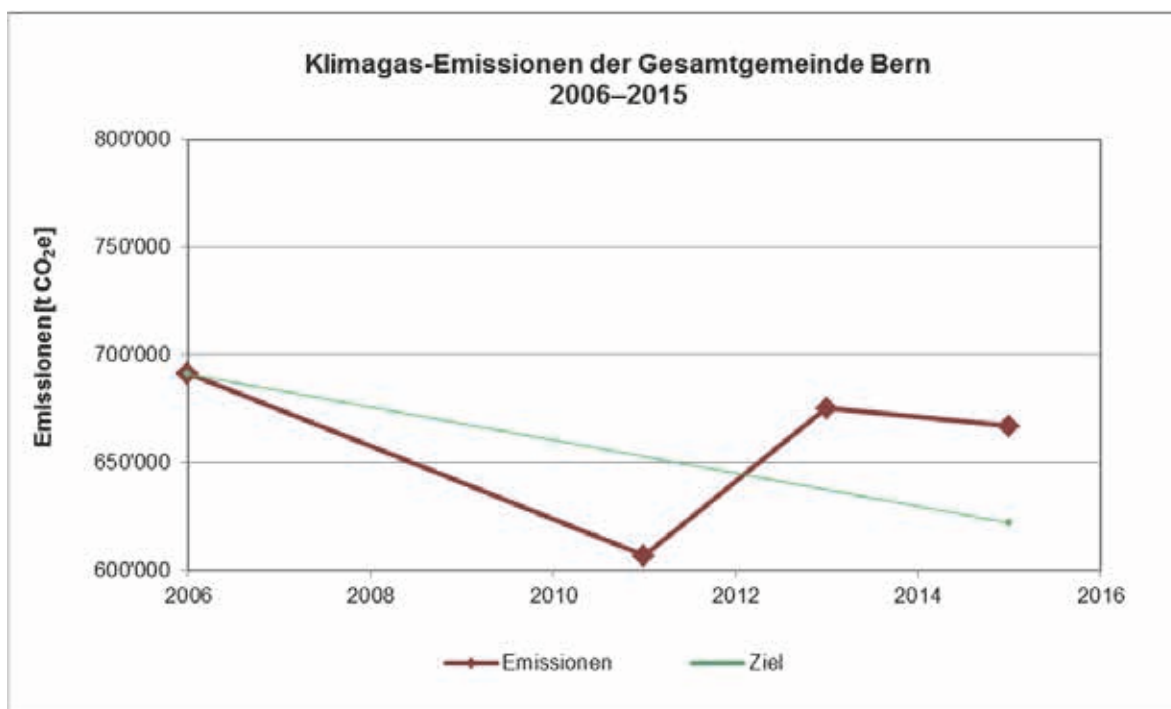
Abbildung 26: Vergleich der Entwicklung des CO 2 e-Ausstosses der Gesamtgemeinde Bern mit der Zielvorgabe (Quelle: Klimagasbilanz der Stadt Bern 2015 [8])
