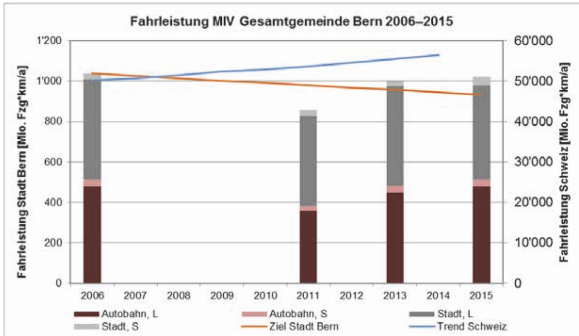
Abbildung 35: Fahrleistung des motorisierten Individualverkehrs. (Quellen: Klimagasbilanzen der Stadt Bern 2011, 2013 und 2015 und BFS – Leistungen des Personenverkehrs (PV-L), Stand Oktober 2015)
