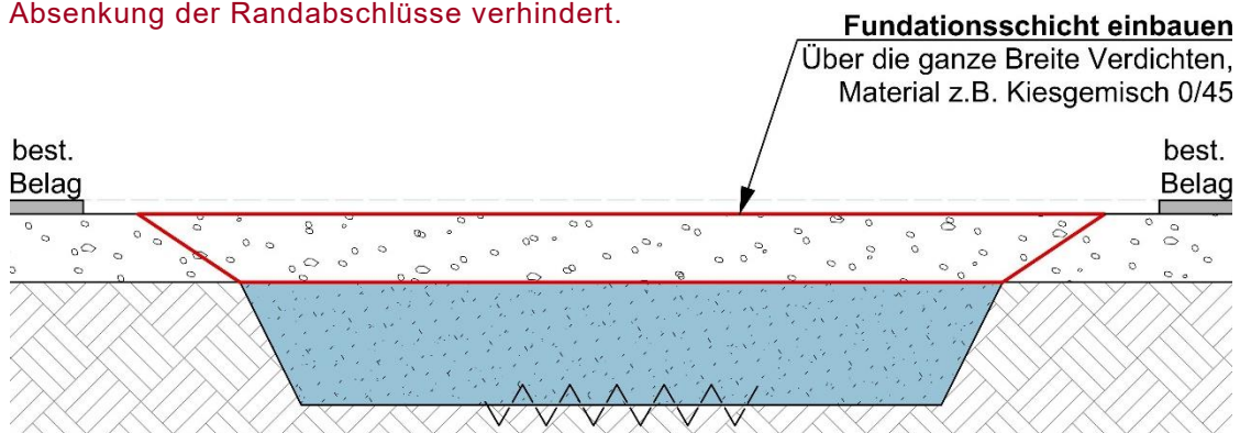
Abbildung 9: Fundationsschicht einbauen, Quelle: Stadtgrün Bern
