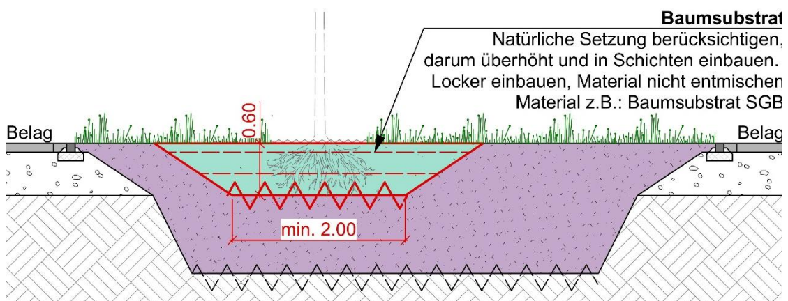
Abbildung 5: Fertigstellung, Quelle: Stadtgrün Bern
