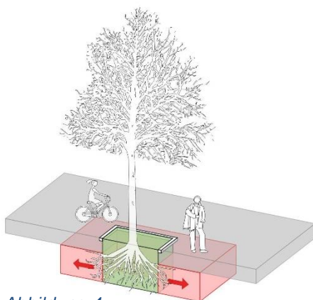
Abbildung 4: Unterirdische Vergrößerung des Wurzelraums unter Belagsflächen Quelle: Stadtgrün Bern
