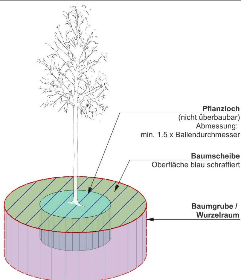
Abbildung 1: Wichtige Begriffe im Zusammenhang mit Strassenbäumen, Quelle: Stadtgrün Bern
