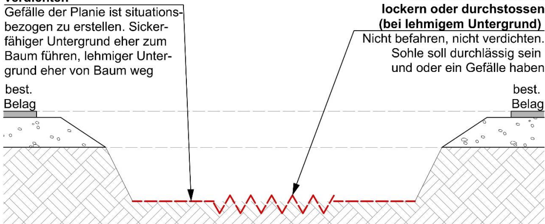
Abbildung 7: Sohle lockern, Quelle: Stadtgrün Bern
