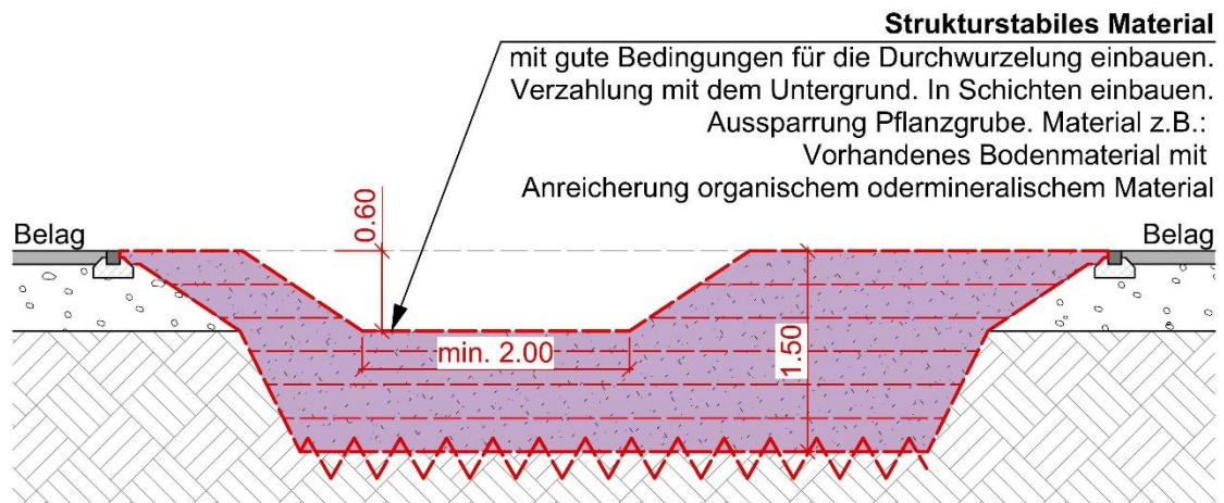
Abbildung 4: Material für Durchwurzelung einbauen, Quelle: Stadtgrün Bern
