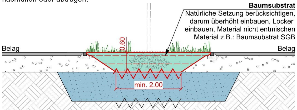
Abbildung 12: Fertigstellung, Quelle: Stadtgrün Bern
