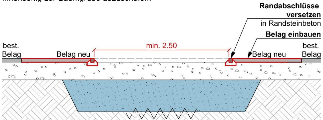
Abbildung 10: Belageinbau und Randabschlüsse, Quelle: Stadtgrün Bern
