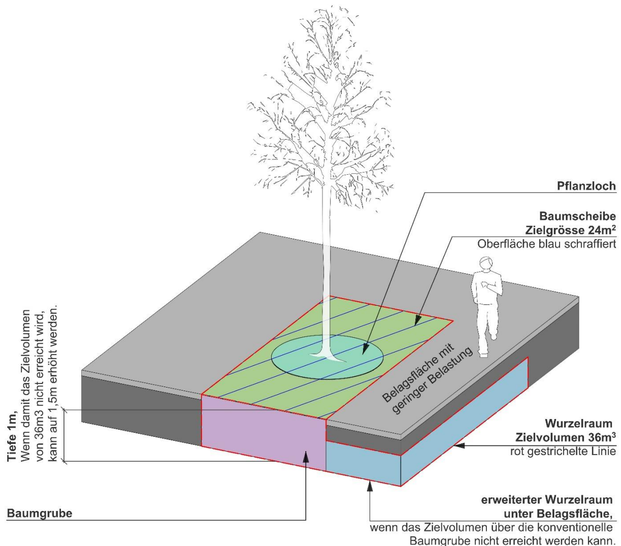
Abbildung 5: Anforderungen Wurzelraum, Quelle: Stadtgrün Bern
