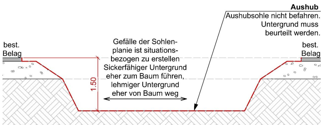
Abbildung 1: Aushub, Quelle: Stadtgrün Bern
