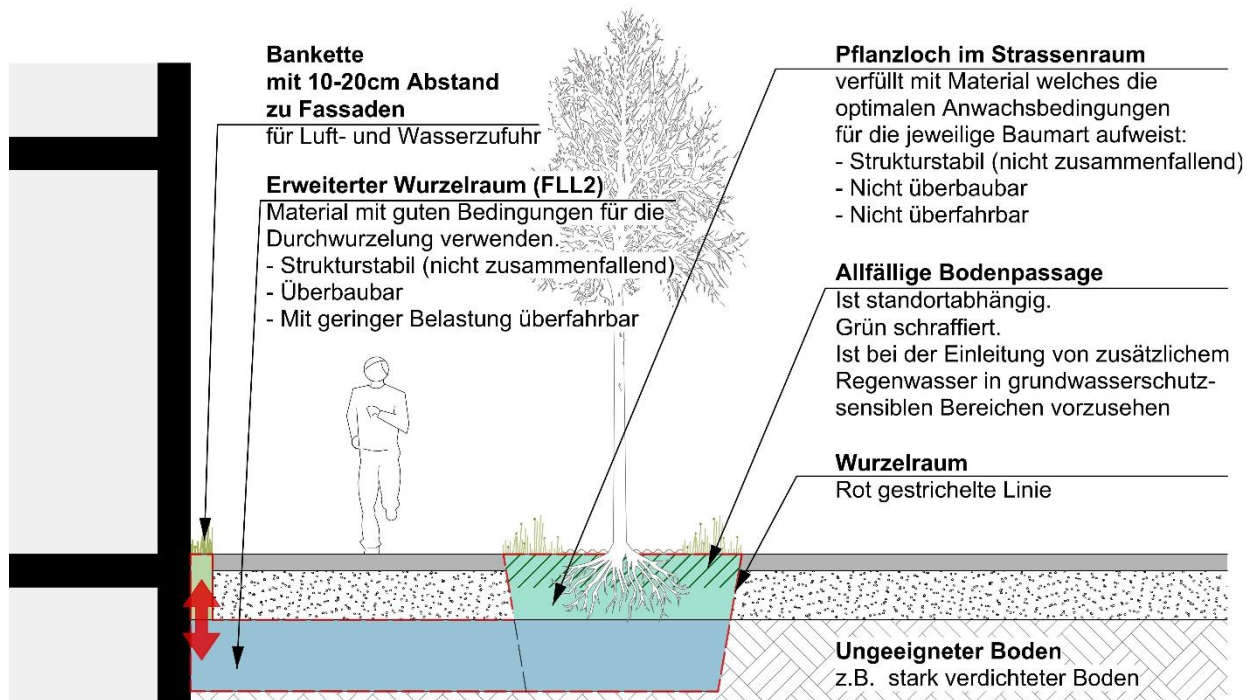
Abbildung 12: Vergrößerung des Wurzelraums zu einer Hausfassade hin. Verwendung von überbaubarem Substrat (Zielgröße Wurzelraum 36 m³ = rot gestrichelte Linie). Quelle: Stadtgrün Bern
