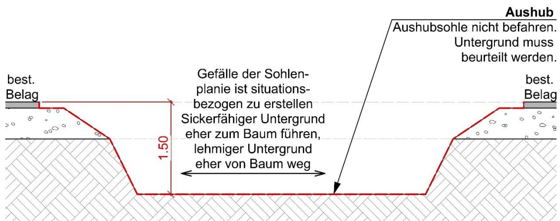
Abbildung 6: Aushub, Quelle: Stadtgrün Bern
