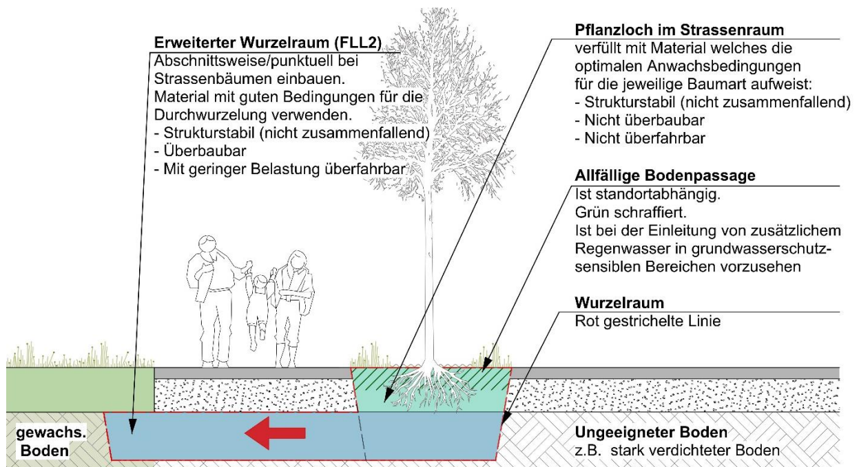
Abbildung 11: Wurzelbrücke zur Schaffung eines vergrösserten Wurzelraumes. Vergrösserung des Wurzelraums mit überbaubarem Substrat (Zielvolumen 36 \text{ m}^3 = rot gestrichelte Linie). Quelle: Stadtgrün Bern
