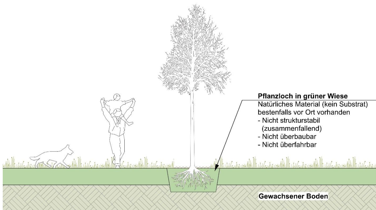
Abbildung 8: Schematische Skizze des Szenarios 1, Quelle: Stadtgrün Bern
