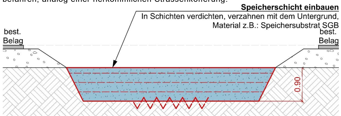
Abbildung 8: Speicherschicht einbauen, Quelle: Stadtgrün Bern
