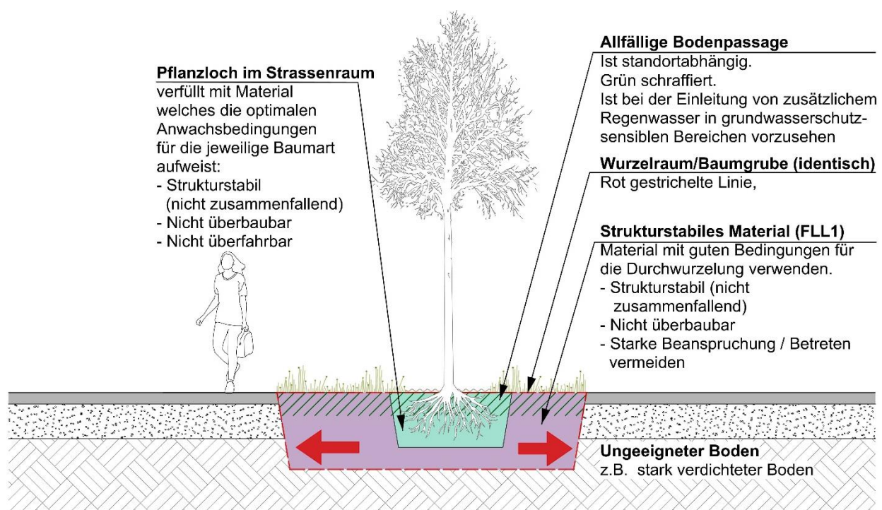
Abbildung 9: Schematische Skizze des Szenarios 2: nicht überbaubar, aber strukturstabil mit einem Wurzelraum (rot gestrichelt) von 36 m 3 . Quelle: Stadtgrün Bern
