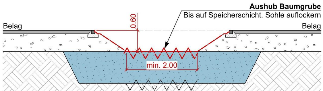
Abbildung 11: Aushub Baumgrube, Quelle: Stadtgrün Bern
