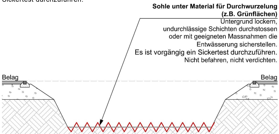
Abbildung 3: Sohle lockern, Quelle: Stadtgrün Bern
