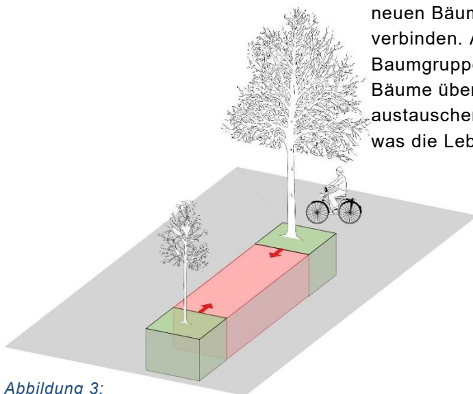
Abbildung 3: Verbindung von Wurzelräumen Quelle: Stadtgrün Bern
