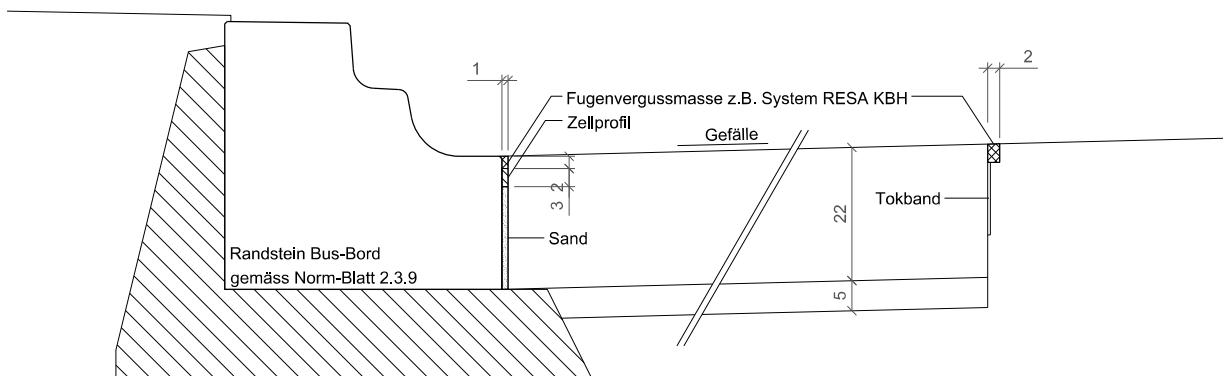
Detail Randabschluss 1: 10
