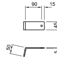
DETAIL 3 Gedübelte Ausführung
