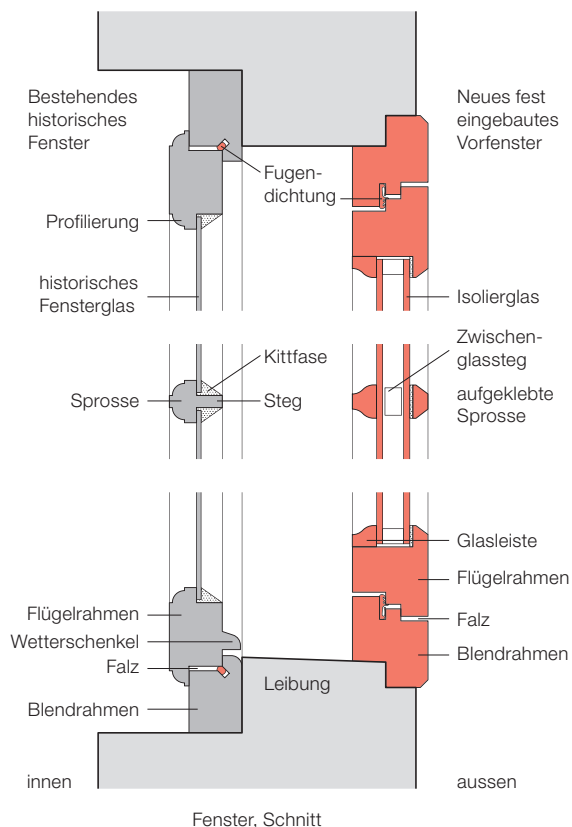
Fenster, Schnitt
