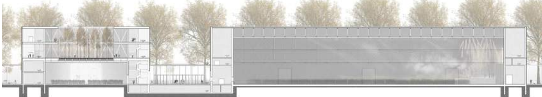
Längsschnitt
