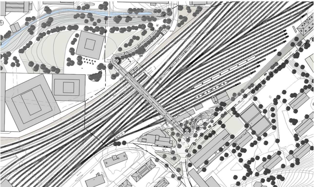
Abbildung 10: Passerelle Fuss- und Veloverkehr, Siegerprojekt Scursun (Team Fürst Laffranchi Bauing. GmbH 2020)
