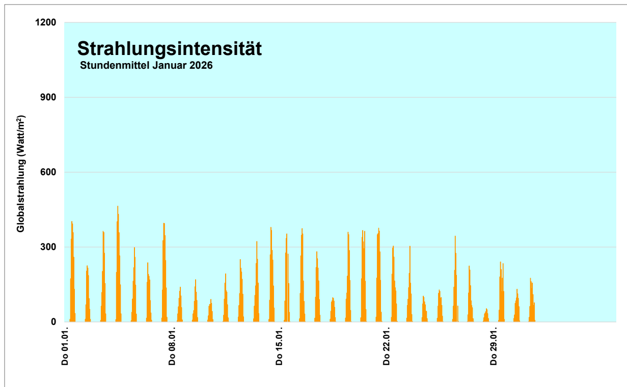
Abbildung 1: Strahlungsintensität, Bern Morgartenstrasse, Januar 2026
