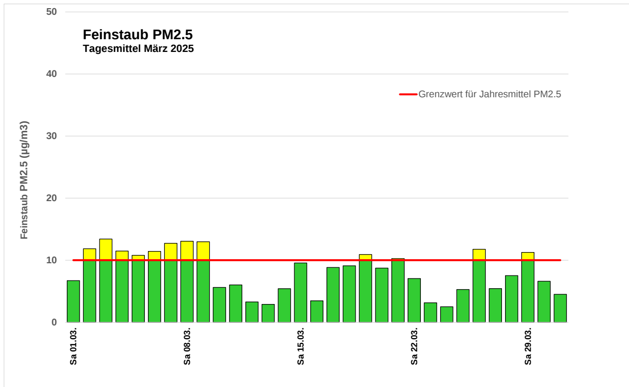
Abbildung 4: Feinstaub PM2.5, Bern Morgartenstrasse, Tagesmittel März 2025
