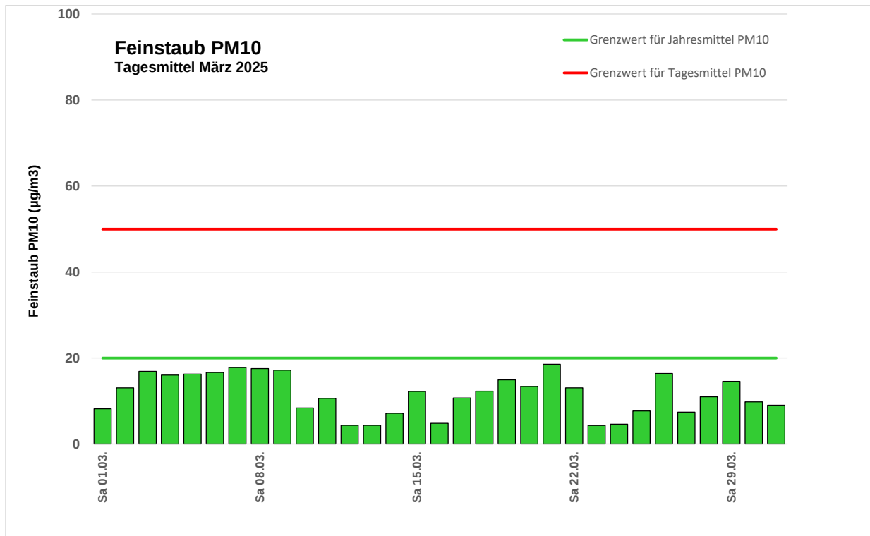
Abbildung 3: Feinstaub PM10, Bern Morgartenstrasse, Tagesmittel März 2025
