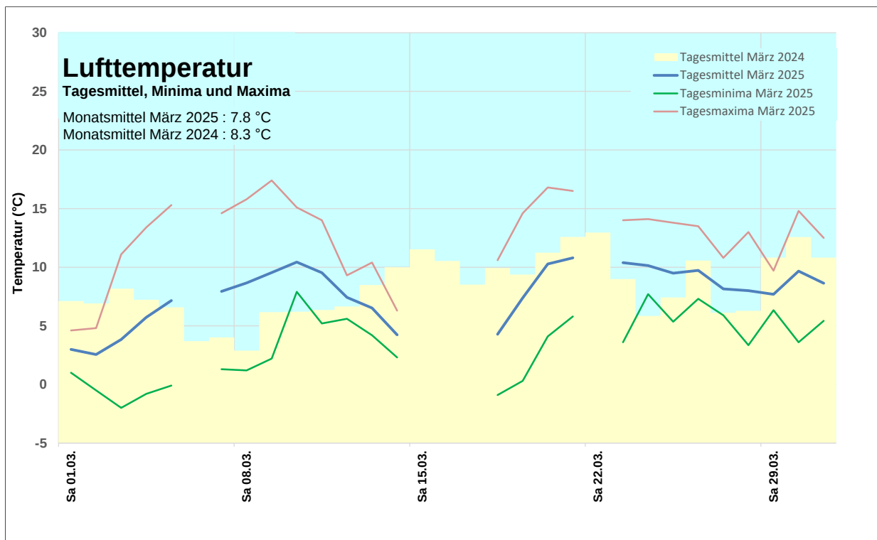
Abbildung 1: Lufttemperatur Bern Morgartenstrasse März 2025
