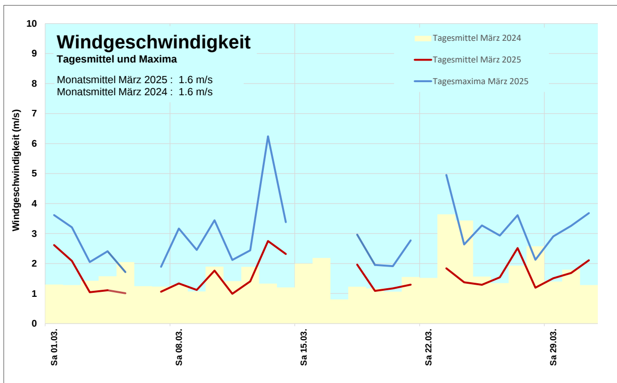
Abbildung 4: Windgeschwindigkeit, Bern Morgartenstrasse, März 2025
