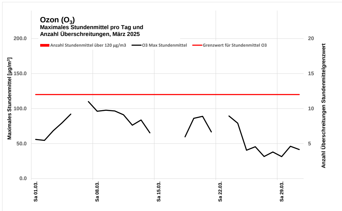
Abbildung 2: Ozon, Bern Morgartenstrasse, maximales Stundenmittel pro Tag und Anzahl Überschreitungen, März 2025
