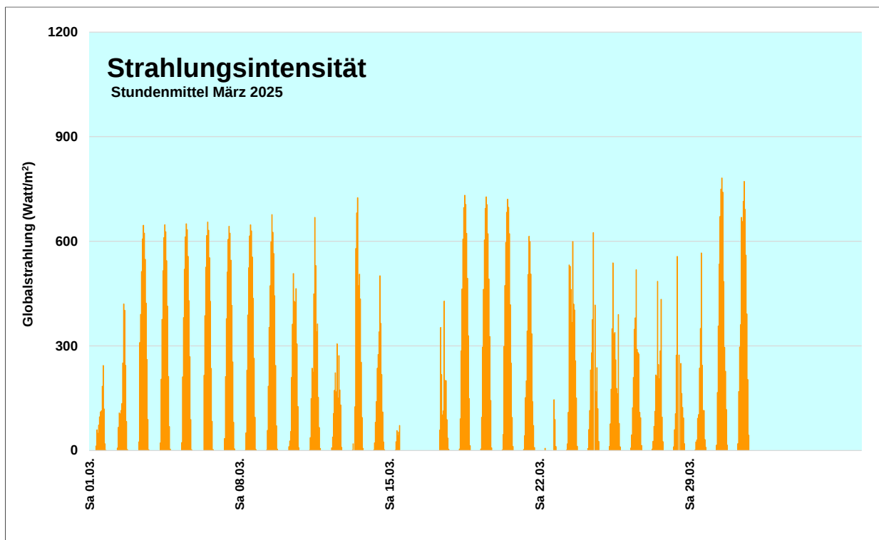
Abbildung 2: Strahlungsintensität, Bern Morgartenstrasse, März 2025
