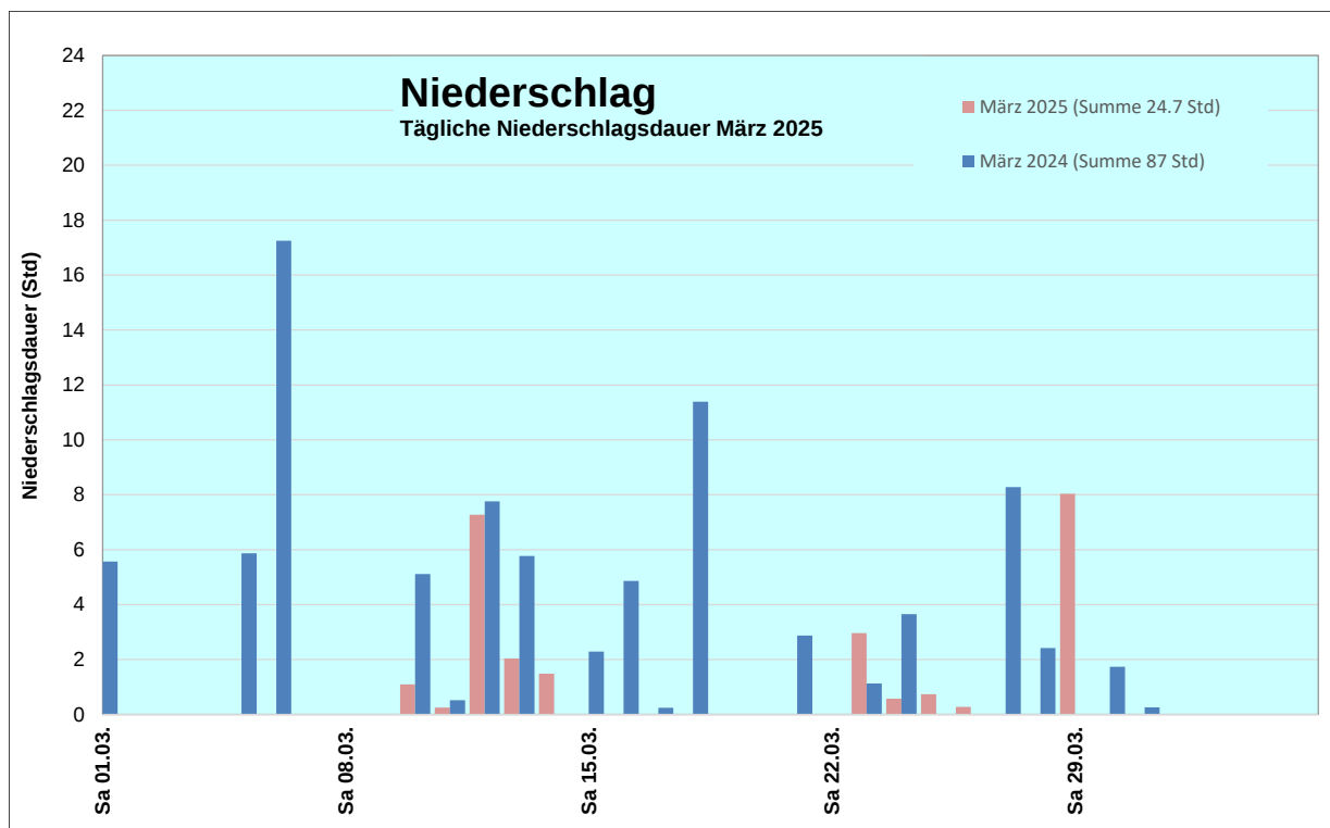
Abbildung 3: Niederschlag, Bern Morgartenstrasse, März 2025
