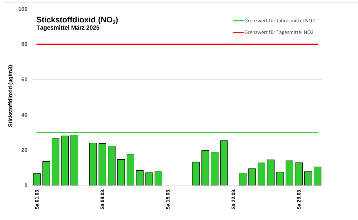
Abbildung 1: Stickstoffdioxid (NO 2 ), Bern Morgartenstrasse, Tagesmittel März 2025
